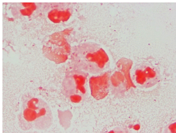
(Hucker変法 1,000倍)
